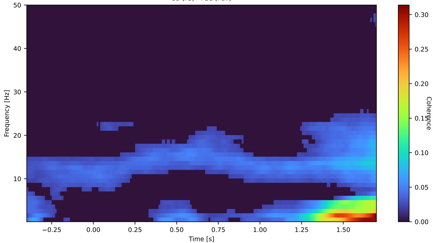
8B (F3) - PEC (P17)
